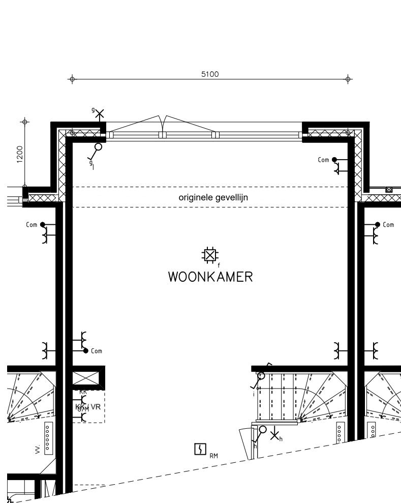
UITBOUW 1,2 METER BNR 6 t/m 11
