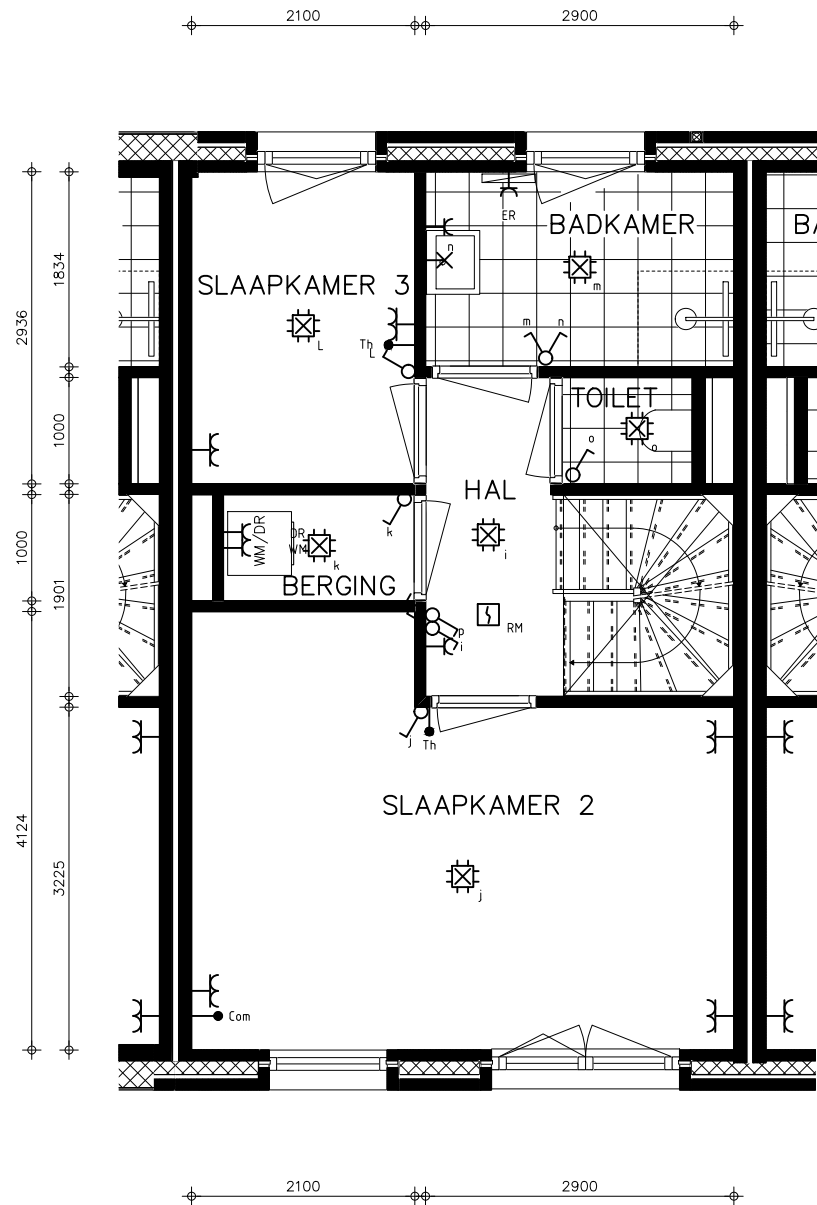
bouwnummer 10 1E VERDIEPING
