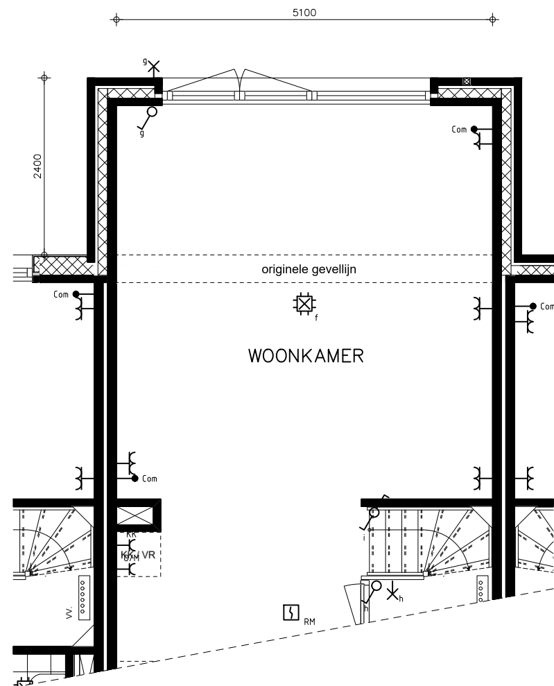
UITBOUW 2,4 METER BNR 6 t/m 11
