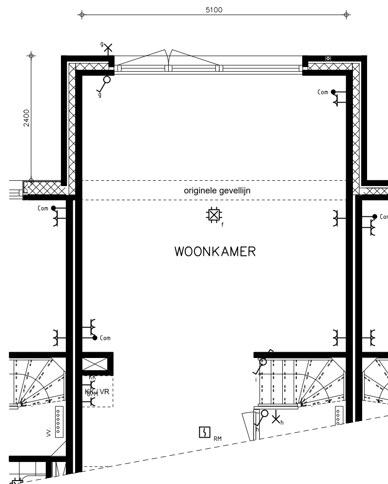
UITBOUW 2,4 METER BNR 6 t/m 11
