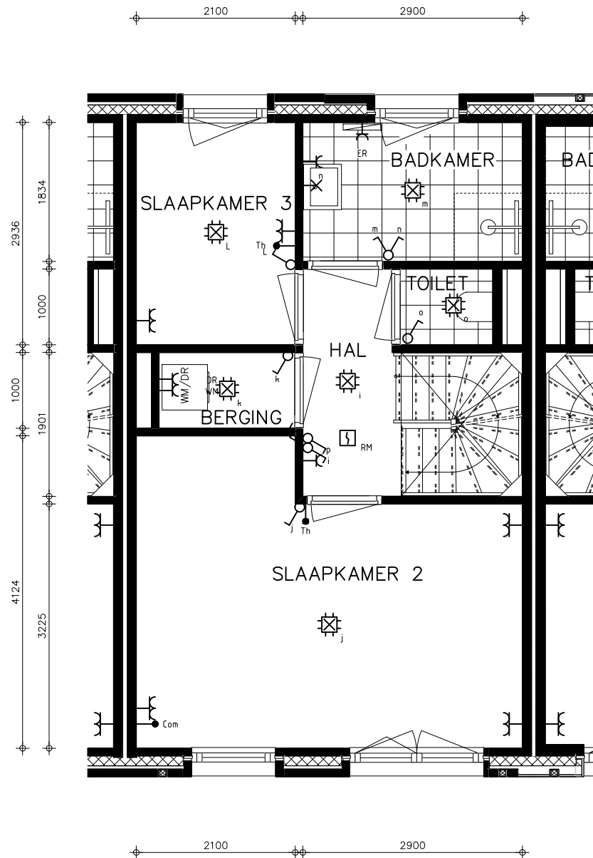
bouwnummer 07 1E VERDIEPING
