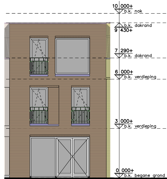
bouwnummer 07 OOSTGEVEL
