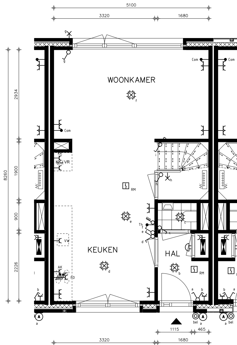
bouwnummer 07 BEGANE GROND
