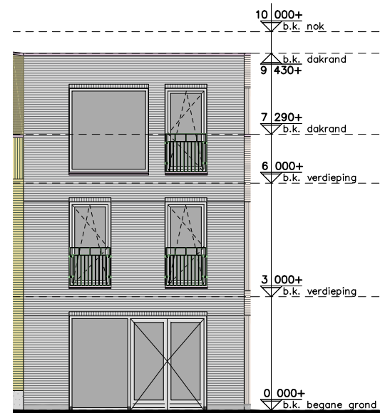
bouwnummer 09 OOSTGEVEL
