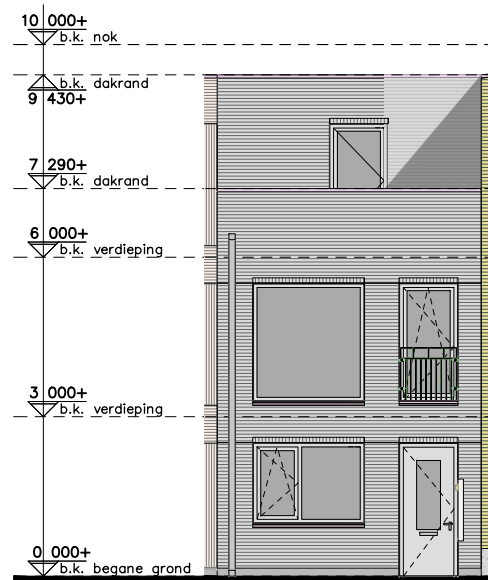
bouwnummer 09 WESTGEVEL
