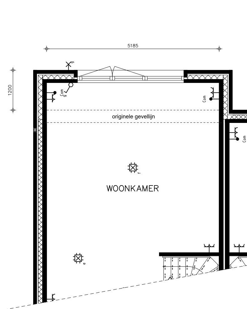
UITBOUW 1,2 METER BNR 12&13
