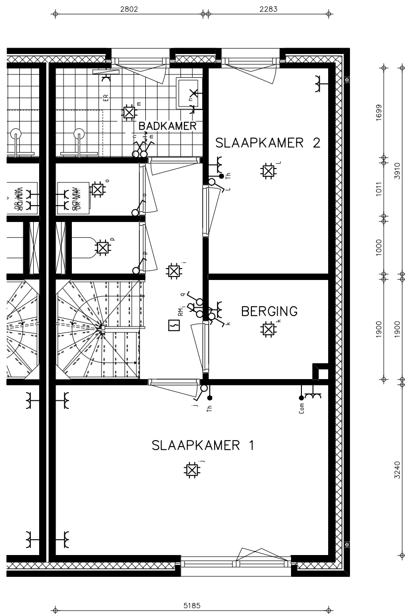
bouwnummer 12 1E VERDIEPING
