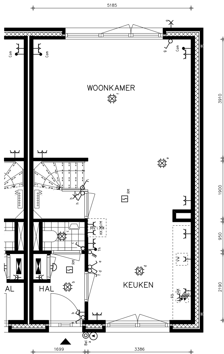
bouwnummer 12 BEGANE GROND
