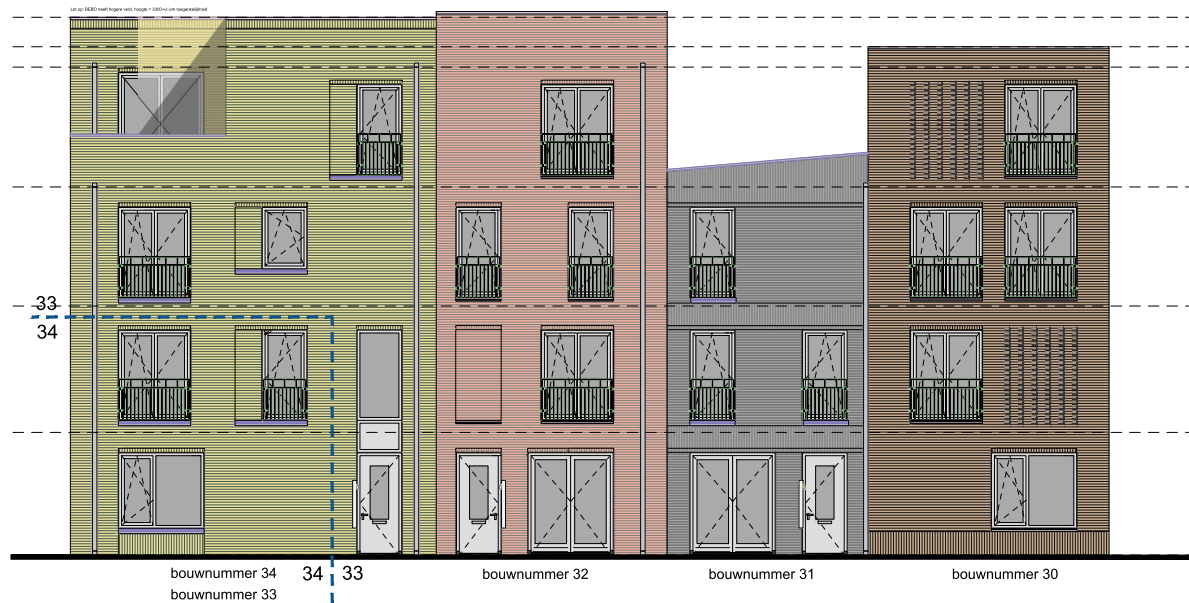
OOSTGEVEL
