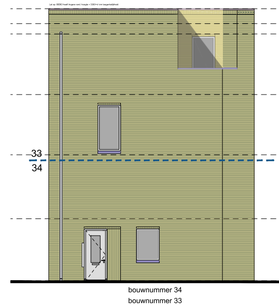
ZUIDGEVEL
