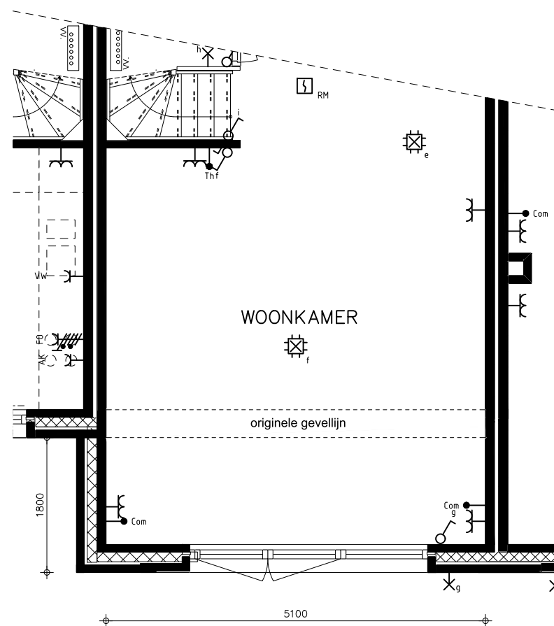
UITBOUW 1,8 METER BNR 36
