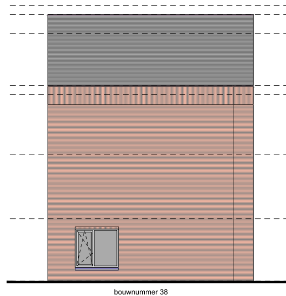
ZUIDGEVEL
