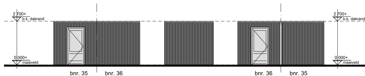
PRINCIPE AANZICHTEN voor werkelijke vorm zie situatietekening
