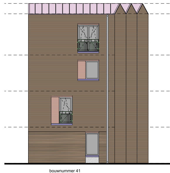
ZUIDGEVEL
