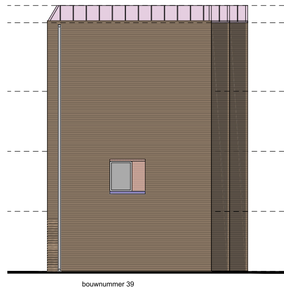
NOORDGEVEL
