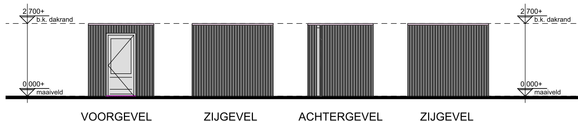
PRINCIPE AANZICHTEN voor werkelijke vorm zie situatietekening
