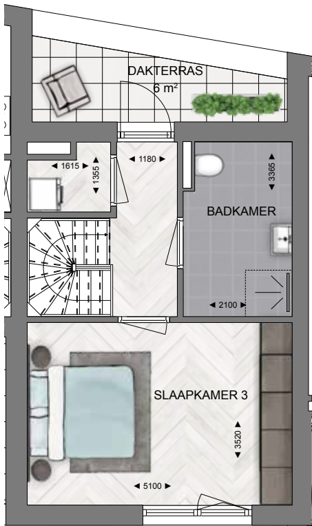
3 E VERDIEPING
